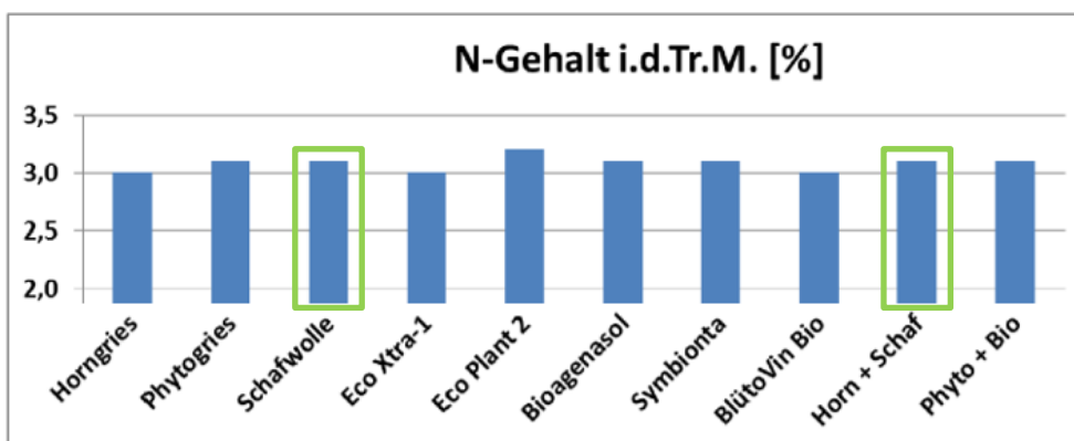
Abb. 8: Stickstoffgehalt in der Trockenmasse zu Versuchsende in Abhängigkeit der unterschiedlichen Düngervarianten bei Teilbevorratung
