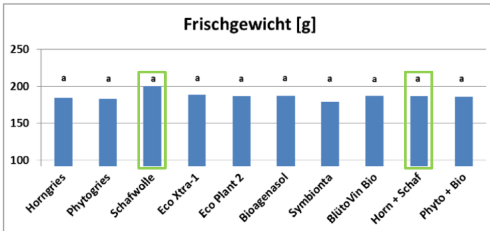
Abb. 7: Frischgewicht der oberirdischen Pflanzenmasse in Abhängigkeit der unterschiedlichen Düngervarianten bei Teilbevorratung, gleiche Buchstaben bedeuten keine signifikanten Unterschiede (Tukey, \alpha < 0,05 ).
